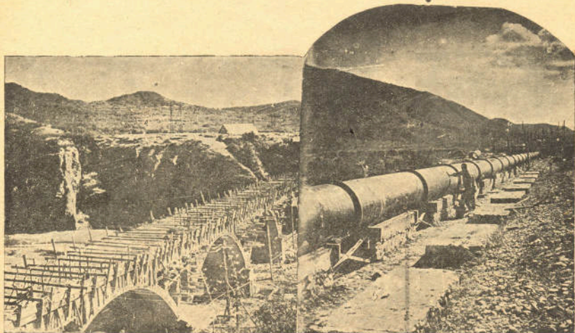
ნატახტარის წყალსადენი. ხიდი რომლის ქვეშაც გადის წყლის მილი. მთავარი მილი
