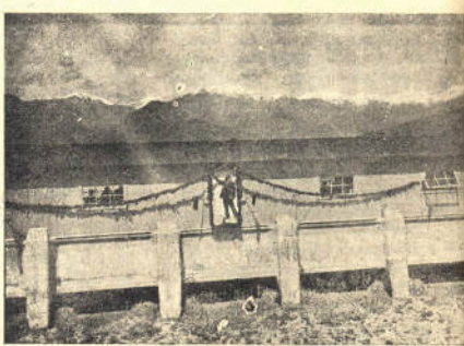
ალაზნის არხის მთავარი საგებარე წყლის გაშენების დროს.
