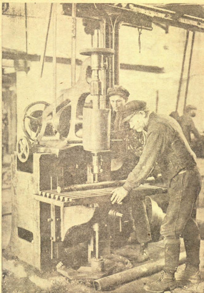
გ ა თ მ მ ი — გამოცდილი მუშა-ტექნიკოსი მექანიკურ სახელსწრწოში მოწაფეს ასწავლია მანქანაზე მუშაობას
