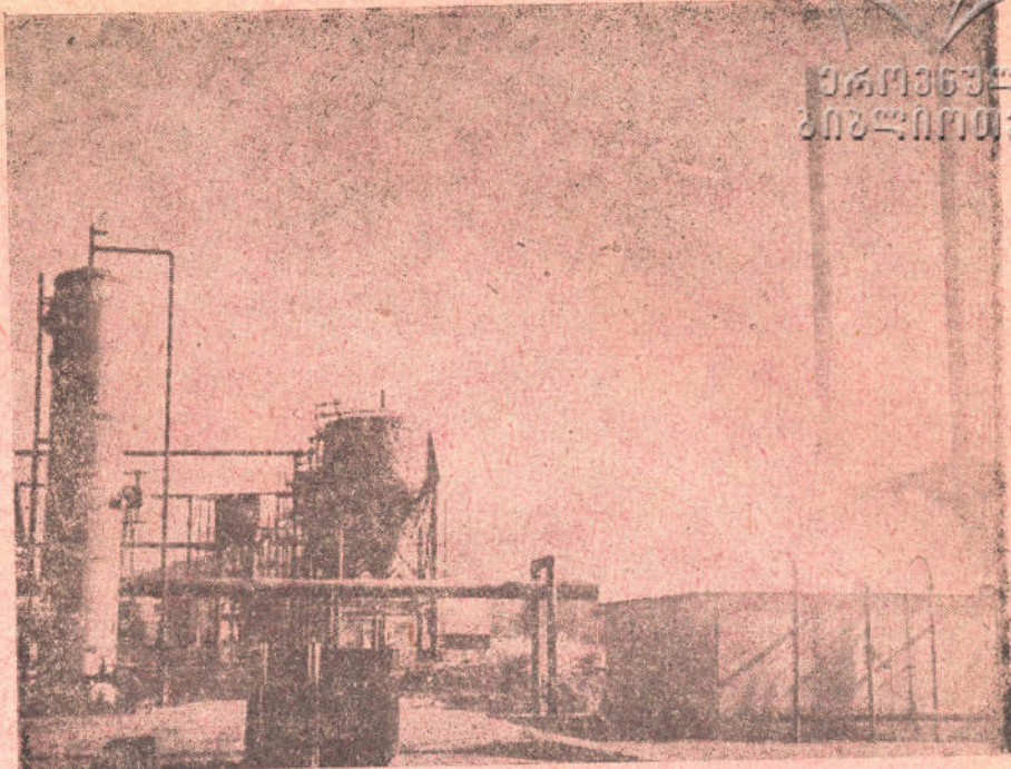
სამ. ნავთი. შირაზანის ნავთის გამოსახდელი ქარხანა.
