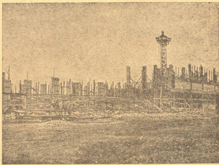
მარცხნივ—ფერო-მარგანცის ქარხნის მუშათა კლუბის მშენებლობა ზესტაფონში, მარჯვნივ—ფერო-მარგანცის ქარხნის საღუმელე კორპუსის მშენებლობა.
