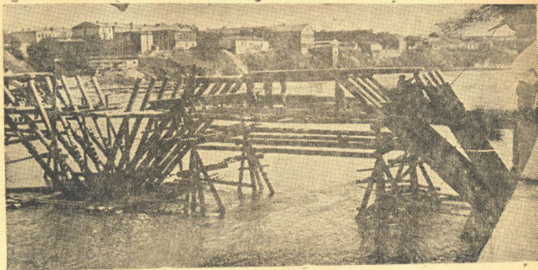
კოზილების დაცემა ბურჯებს შორის
