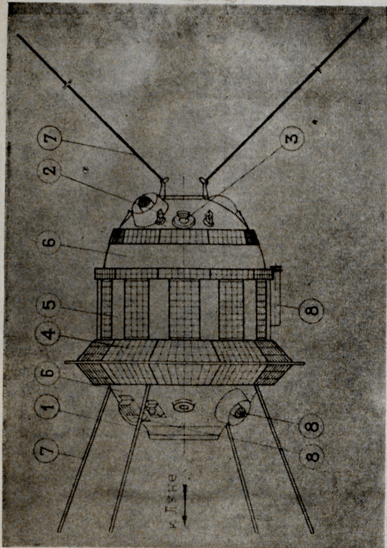
Neste diagrama vemos os principais instrumentos da estação automática interplanetária (Lunik III) com que os soviéticos fotografaram a face oculta da Lua. Os números indicam: 1) iluminador para as câmaras; 2) motor para a orientação do sistema; 3) monitor solar; 4) seção da bateria solar; 5) obturadores do sistema termo-regulador; 6) anteparos térmicos; 7) antenas; 8) dispositivos para pesquisas científicas
