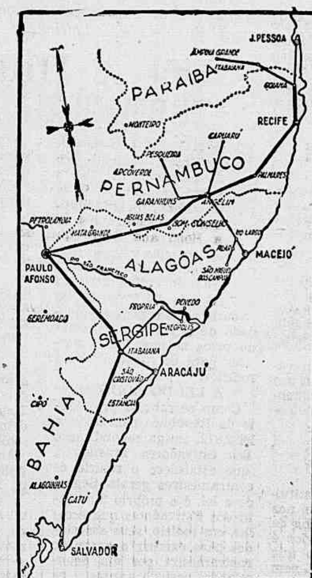
Mapa da zona servida com a energia da Hidrelétrica de São Francisco. Planeja atualmente o governo o aumento da capacidade geradora da usina de Paulo Afonso
